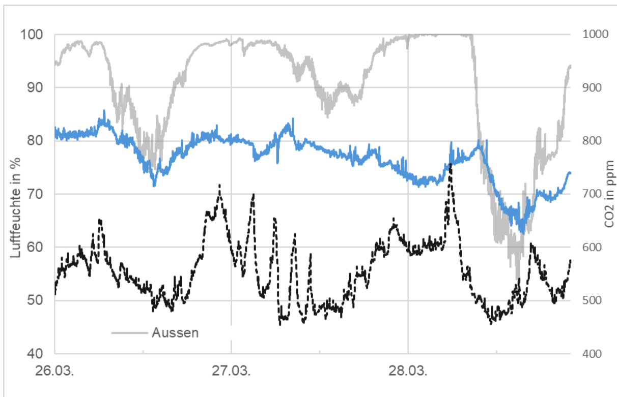
Abbildung 49: Luftfeuchte Außen (grau), in den Boxen A12, A14 und A16 (blau) und CO 2 -Konzentration (durchbrochene Linie) im Stallinneren. NH 3 -Konzentrationen lagen im Messzeitraum im Stallinneren bei 0,4 – 2,4 ppm. Es befanden sich 5 Tiere im Abteil.
