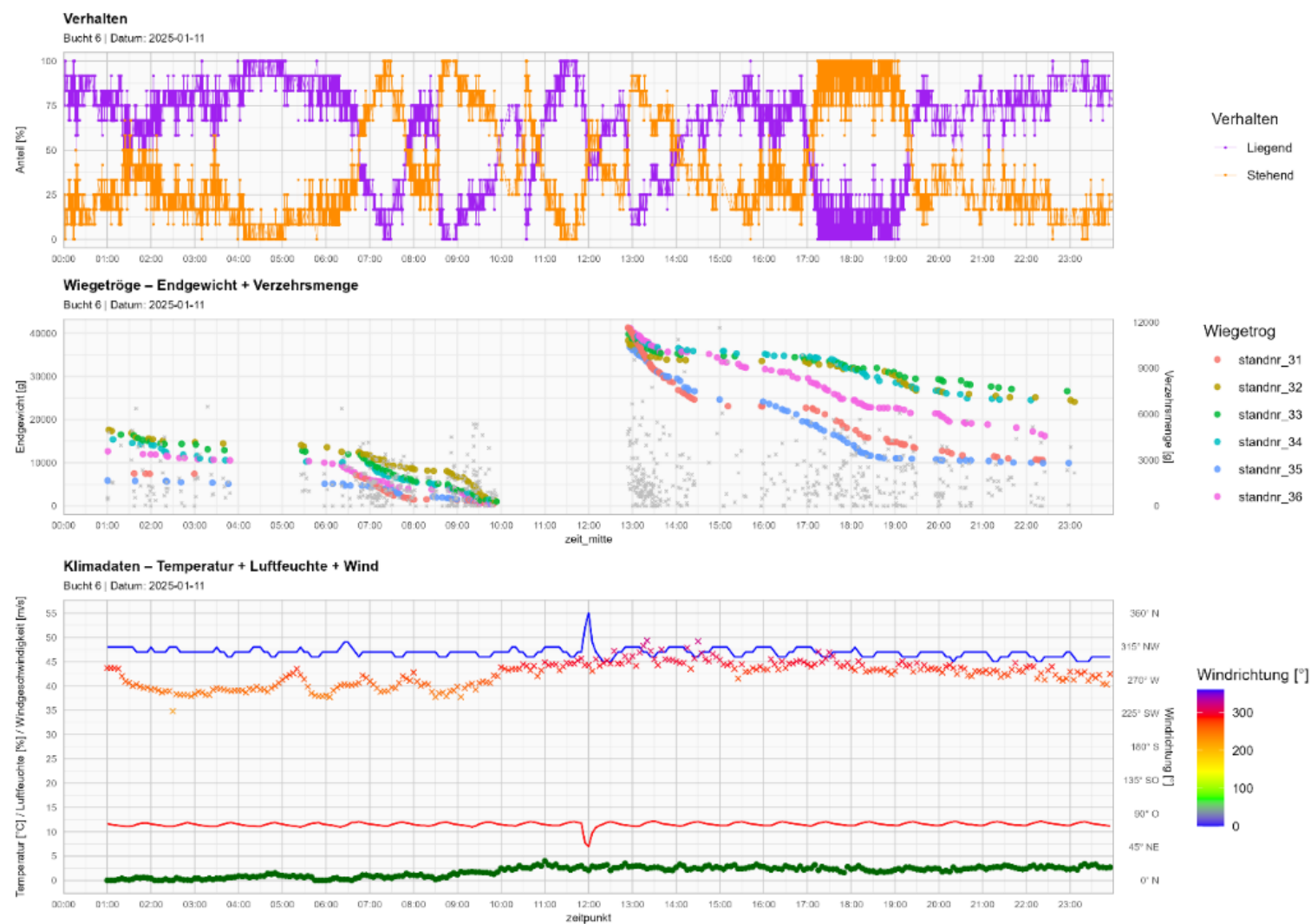
Abbildung 88: Visualisierung von 24 h automatisch generierter Daten aus Bucht 6 (Tretmist) vom 11.01.2025. Oben - Verhaltenswerte (orange - Anteil stehend, lila- Anteil liegend). Mitte - Wiegetrogdaten mit Verzehrmenge und Wiegetrog-Füllstände. Unten - Klimadaten der Stallklimamessungen (grün - Windgeschwindigkeit außerhalb des Stalls, Farbspektrum - Windrichtung außerhalb des Stalls, rot - Temperatur im Stall, und blau – rel. Luftfeuchtigkeit im Stall).
