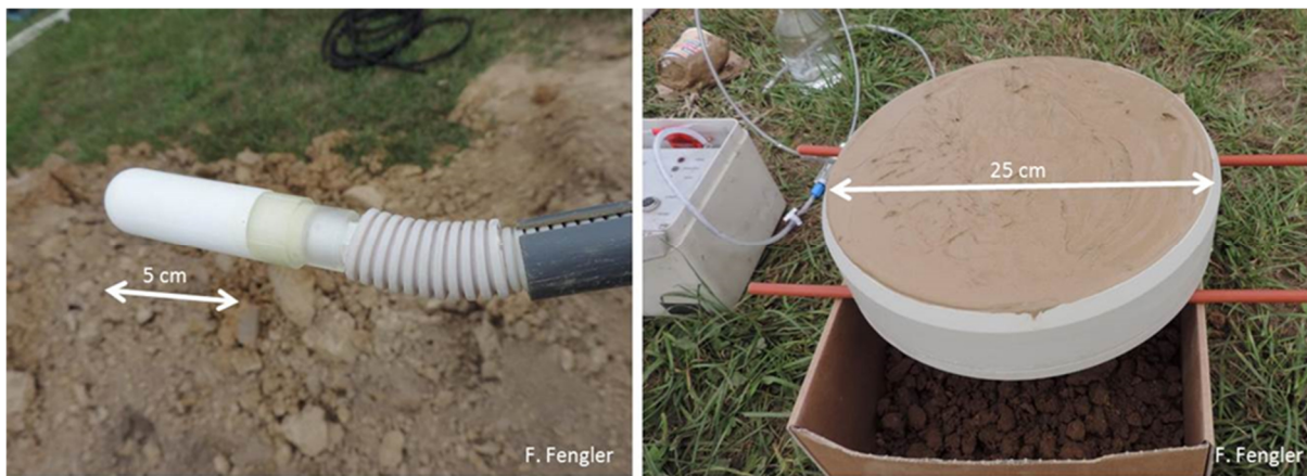
Abbildung 4: Keramik-Saugkerze (links); Saugplatte (rechts)
