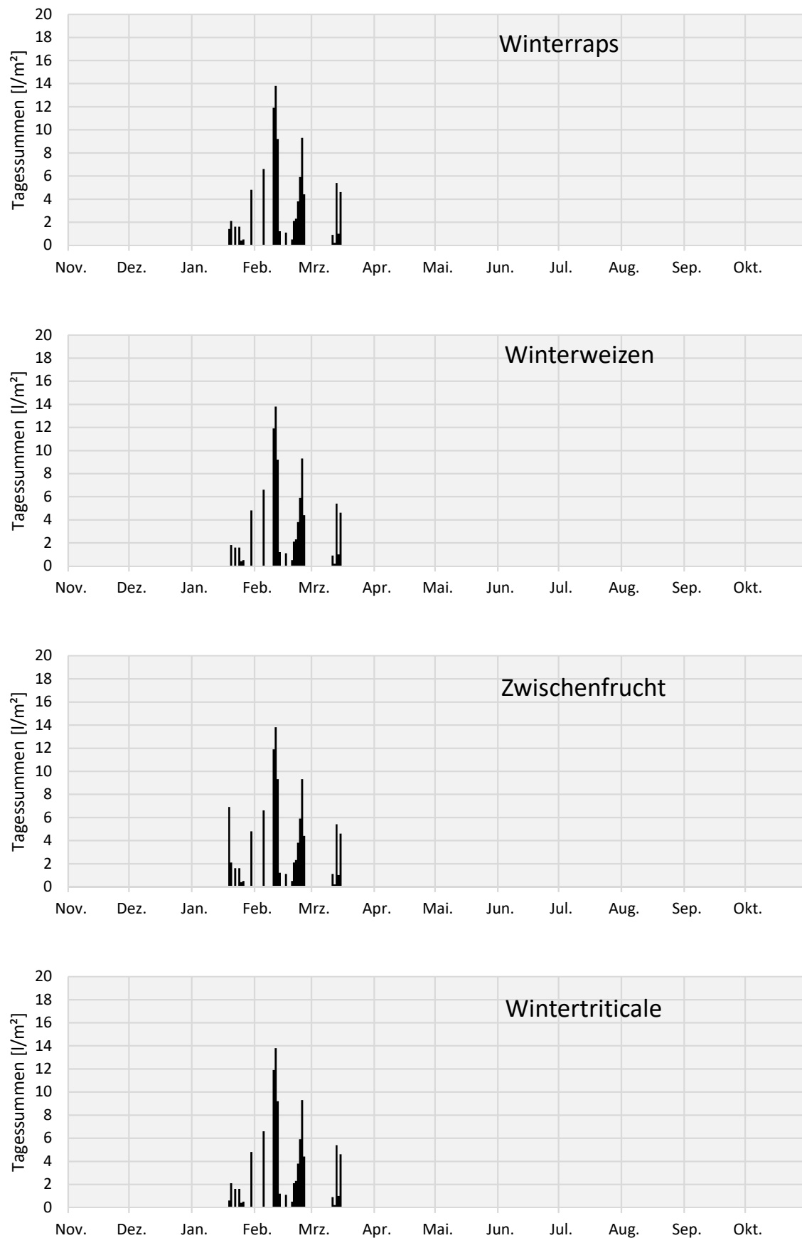
Abbildung 12: Sickerwassermenge der Sickerwasserperiode 2020/21 nach Modell METVER (DWD) in 1m Bodentiefe in Abhängigkeit von der Kulturart
