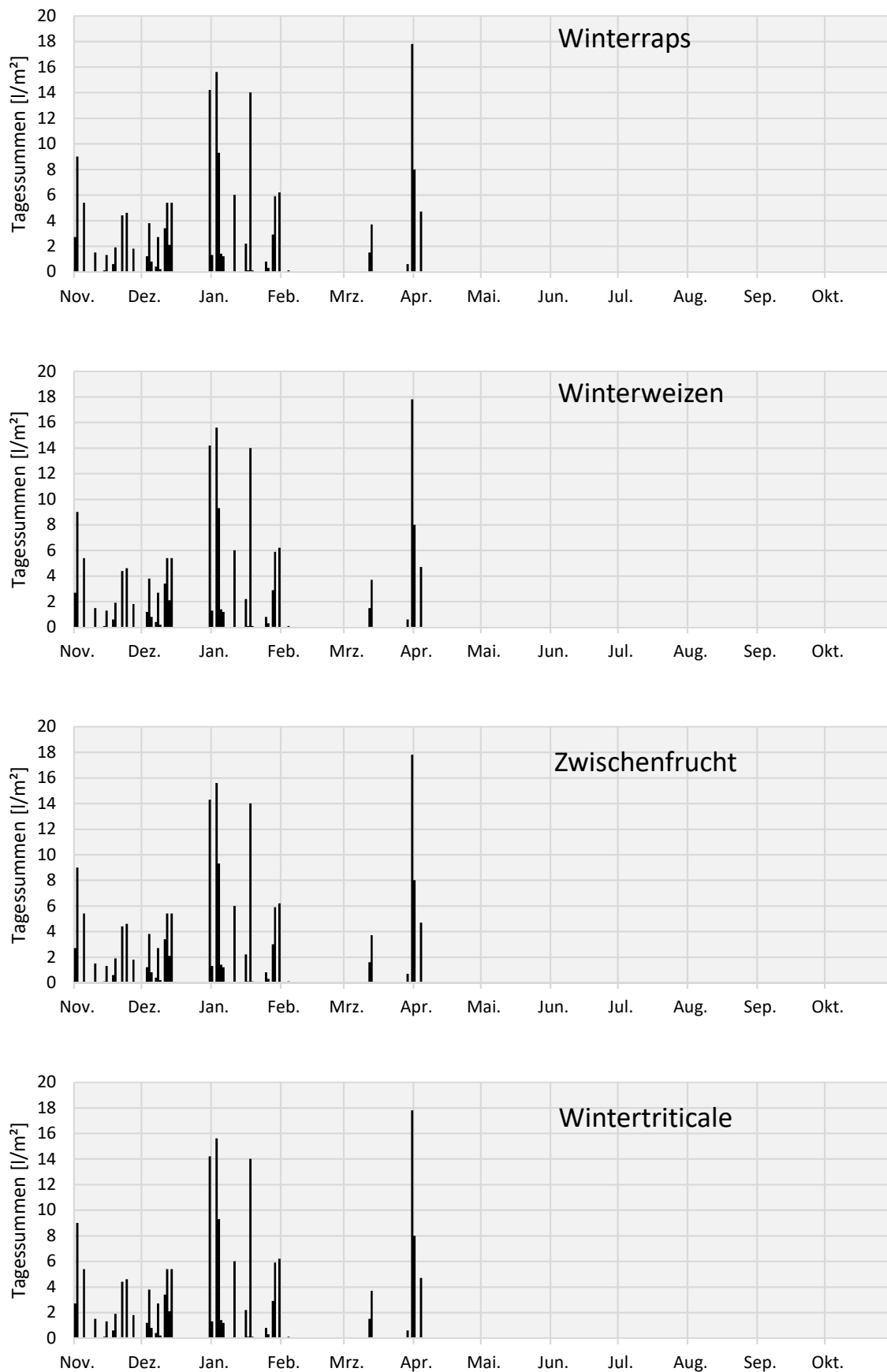
Abbildung 6: Sickerwassermenge der Sickerwasserperiode 2017/18 nach Modell METVER (DWD) in 1m Bodentiefe in Abhängigkeit von der Kulturart
