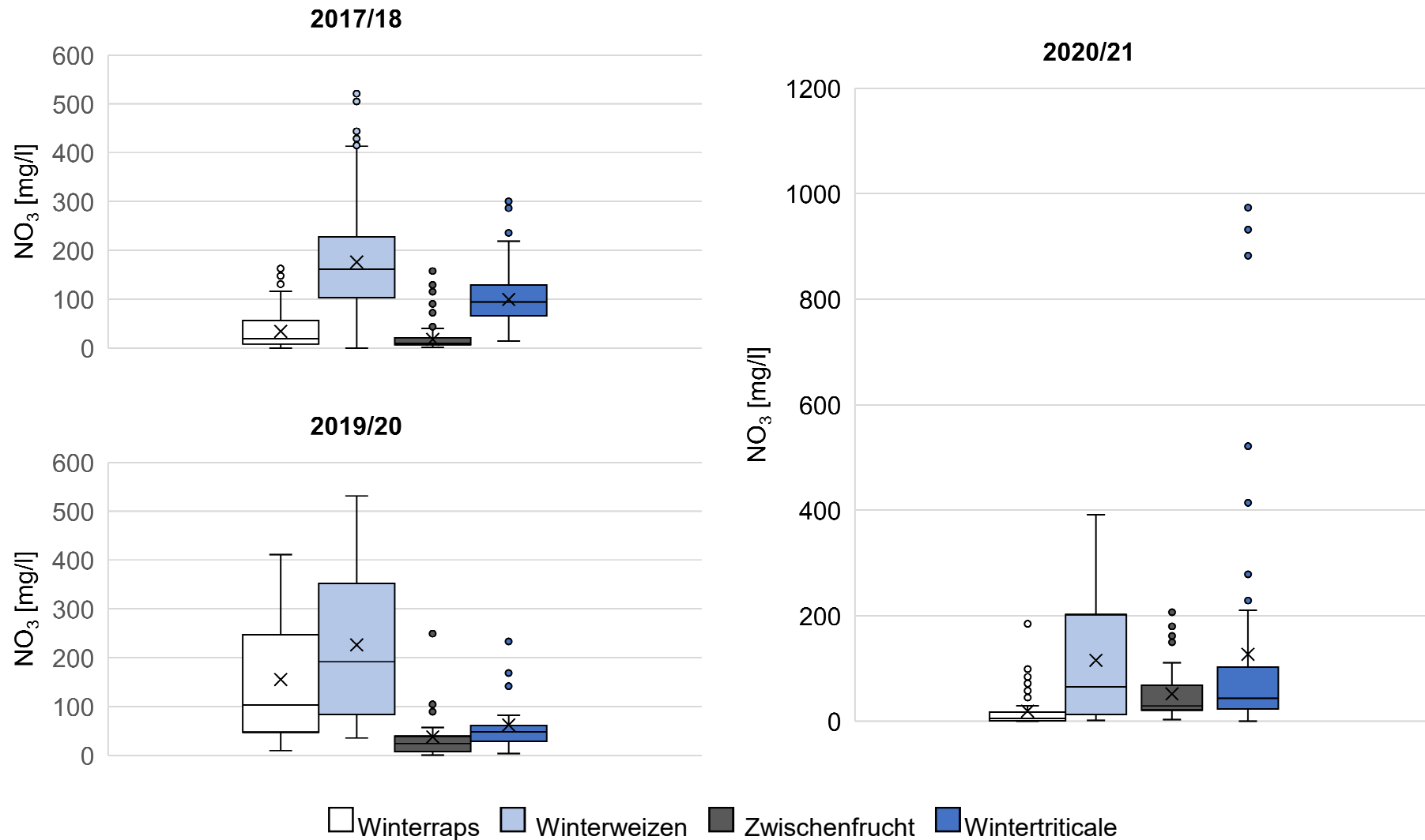
Abbildung 14: Nitratkonzentration im Sickerwasser in 60 cm Bodentiefe während der Sickerwasserperiode in Abhängigkeit von der angebauten Kulturart, Messwerte aller Düngungsvarianten (x=Mittelwert, —=Median, boxplot=Interquartilsabstand, Whisker=1,5-facher Interquartilsabstand, Punkte=Einzelwerte außerhalb des 1,5-fachen Interquartilsabstands), Gülzow 2017-2021
