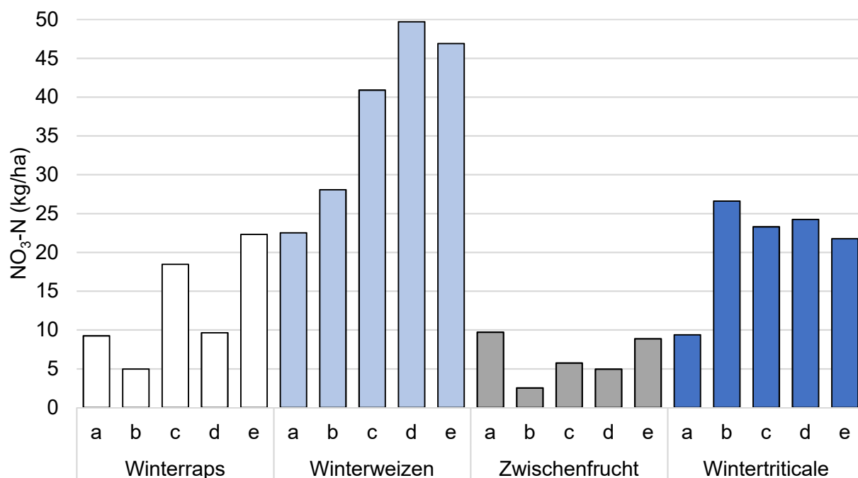
Abbildung 17: Nitrat-Fracht in 60 cm Tiefe während der Sickerwasserperiode in Abhängigkeit von N-Düngung und Kulturart, N-Düngung: a = ohne, b = 80% mineralisch, c = 100% mineralisch, d = 100% organisch-mineralisch nur Frühjahr, e = 100% organisch-mineralisch Herbst und Frühjahr (Mittelwerte 2017-2021)
