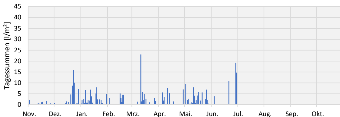
Abbildung 11: Niederschlagsmenge der Sickerwasserperiode 2020/21 (Messwerte, Wetterstation Gülzow bis 30. Juni 2021)
