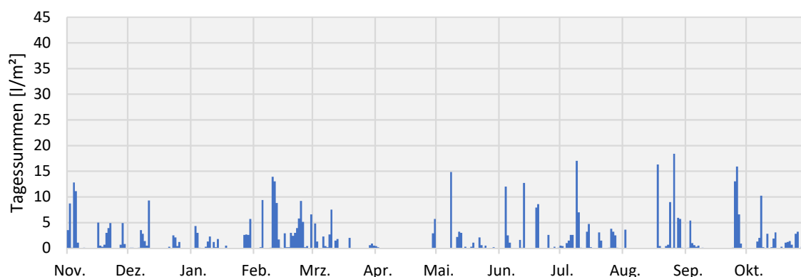
Abbildung 9: Niederschlagsmenge der Sickerwasserperiode 2019/20 (Messwerte, Wetterstation Gülzow)
