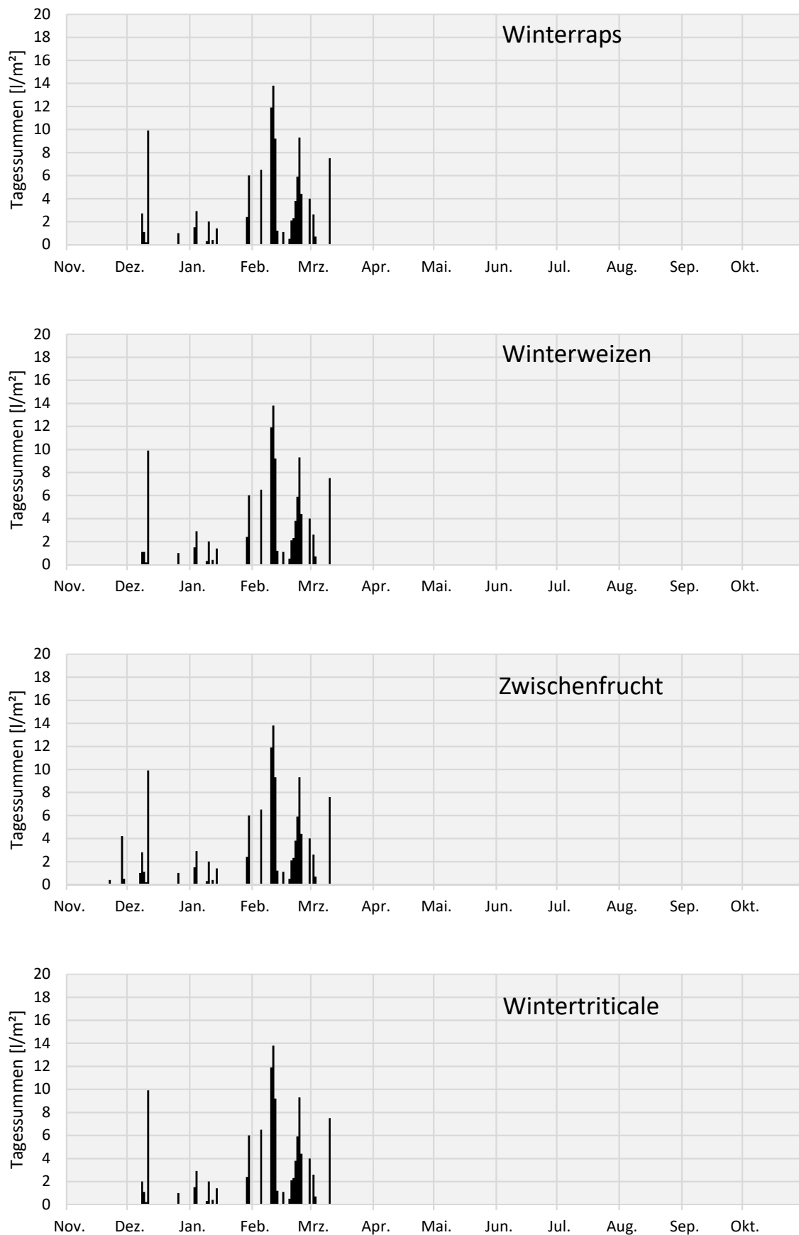
Abbildung 10: Sickerwassermenge der Sickerwasserperiode 2019/20 nach Modell METVER (DWD) in 1m Bodentiefe in Abhängigkeit von der Kulturart
