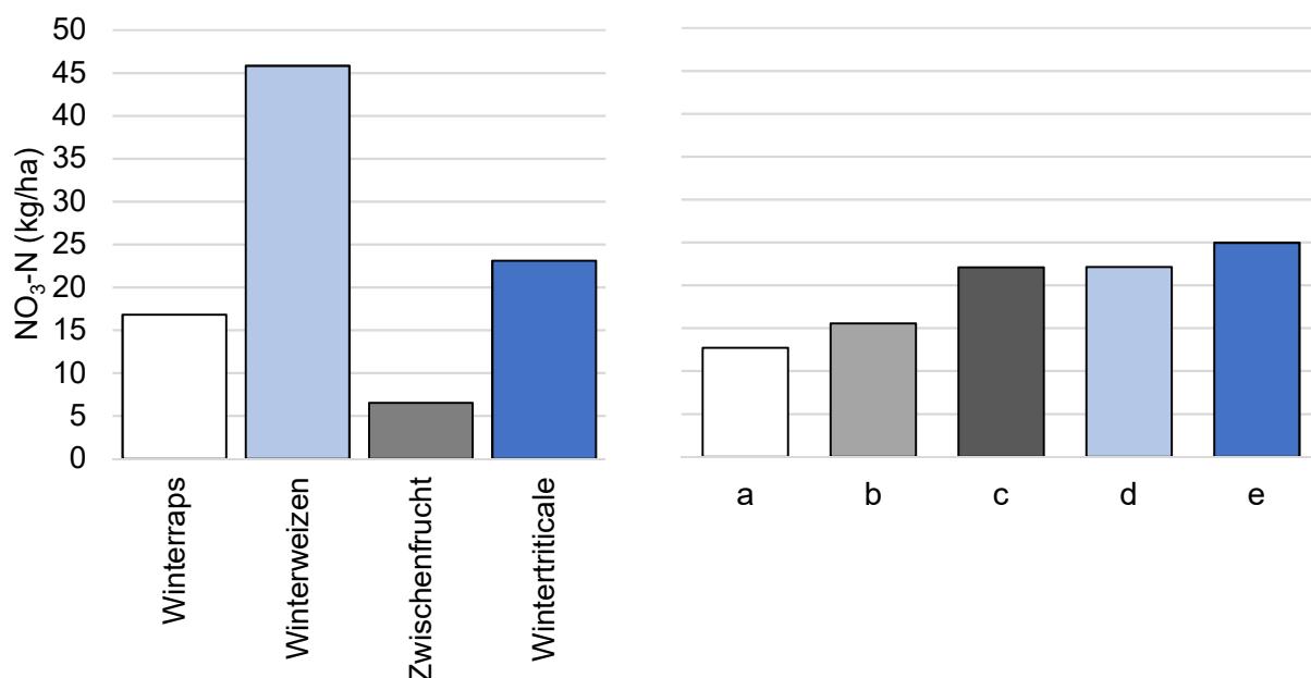
Abbildung 18: Nitrat-Fracht in 60 cm Tiefe während der Sickerwasserperiode in Abhängigkeit von N-Düngung bzw. Kulturart, N-Düngung: a = ohne, b = 80% mineralisch, c = 100% mineralisch, d = 100% organisch-mineralisch nur Frühjahr, e = 100% organisch-mineralisch Herbst und Frühjahr (Mittelwerte 2017-2021)
