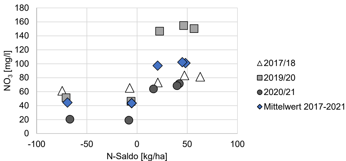
Abbildung 15: Nitratkonzentration (mittlerer Medianwert über die Kulturarten, 60 cm Bodentiefe) in Abhängigkeit vom mittleren N-Saldo der Düngungsvarianten der Fruchtfolge (N-Saldo 2017/18: aus 2 Vorjahren, 2019/20 und 2020/21 aus je 4 Vorjahren, 2017-2021 aus 5 Vorjahren gebildet), Gülzow, 2016-2021
