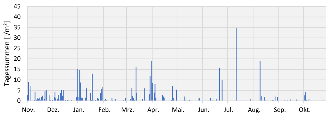
Abbildung 5: Niederschlagsmenge der Sickerwasserperiode 2017/18 (Messwerte, Wetterstation Gülzow)
