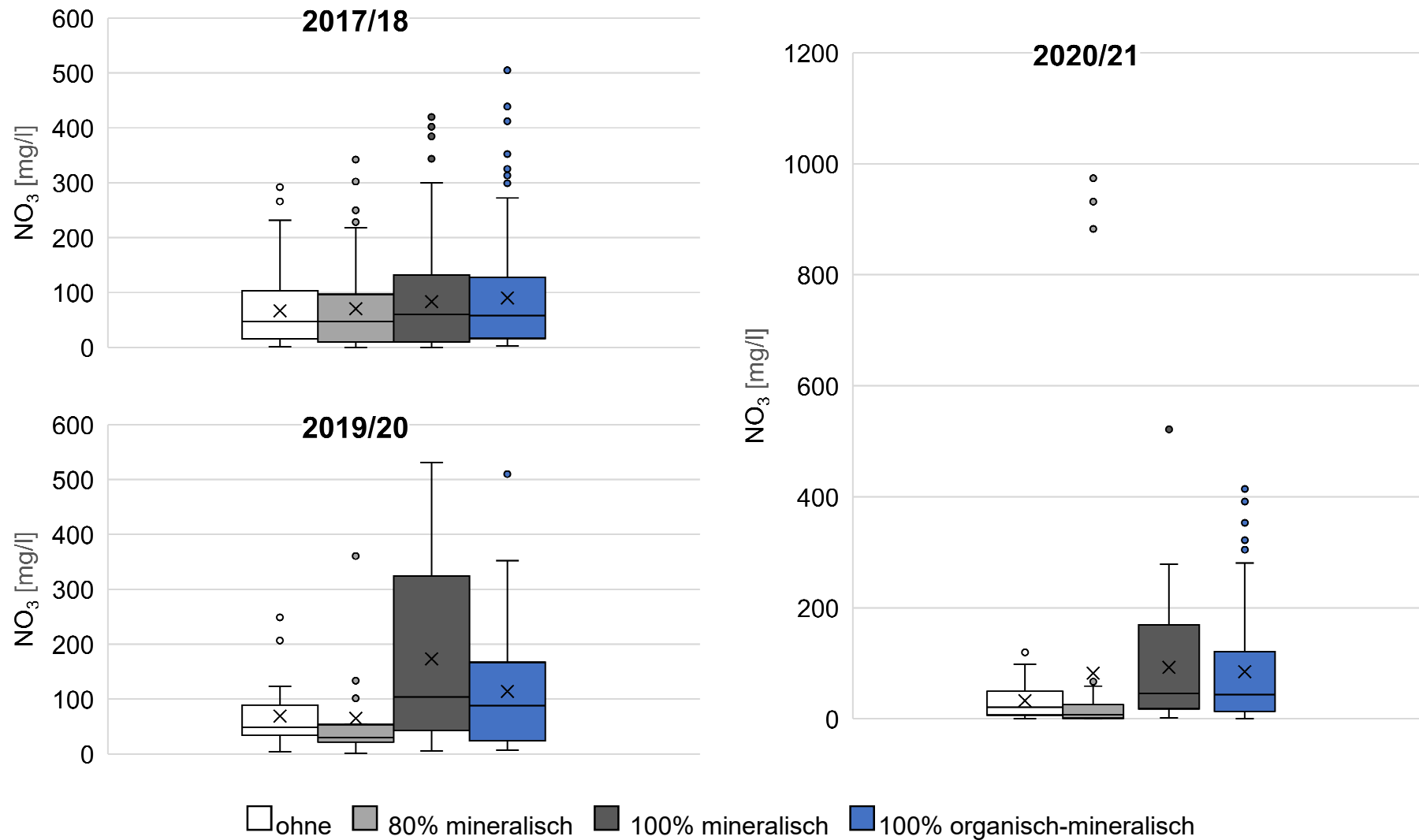
Abbildung 16: Nitratkonzentration im Sickerwasser in 60 cm Bodentiefe während der Sickerwasserperiode in Abhängigkeit von der N-Düngung, Messwerte aller Kulturarten (x=Mittelwert, —=Median, boxplot=Interquartilsabstand, Whisker=1,5-facher Interquartilsabstand, Punkte=Einzelwerte außerhalb des 1,5-fachen Interquartilsabstands), PG 7 und 12 zusammengefasst, Gülzow 2017-2021
