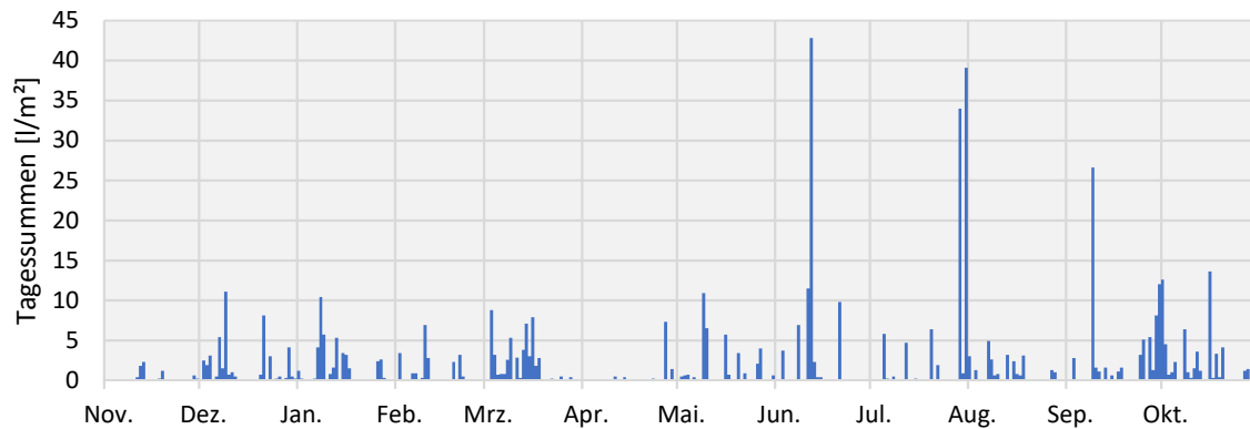
Abbildung 7: Niederschlagsmenge der Sickerwasserperiode 2018/19 (Messwerte, Wetterstation Gülzow)
